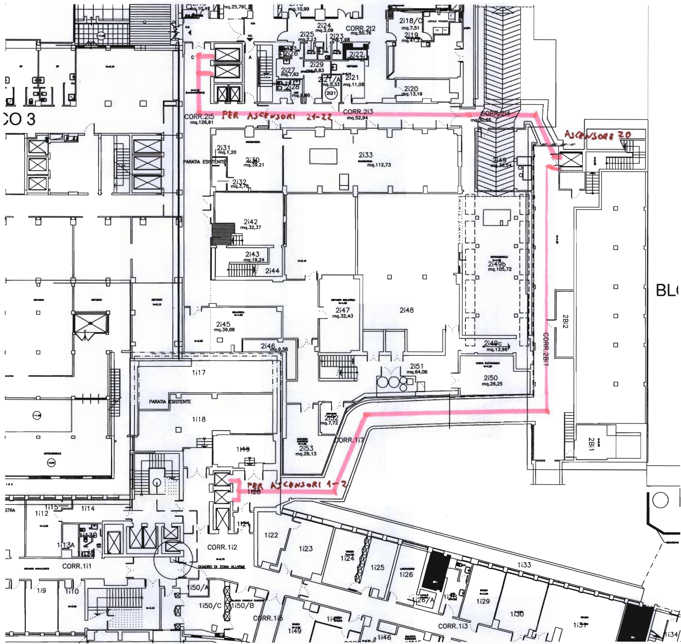
STRALCIO PIANO INTERRATO, PERCORSI DA ASCENSORE 20 AD ASCENSORI 1-2 E 24-22
